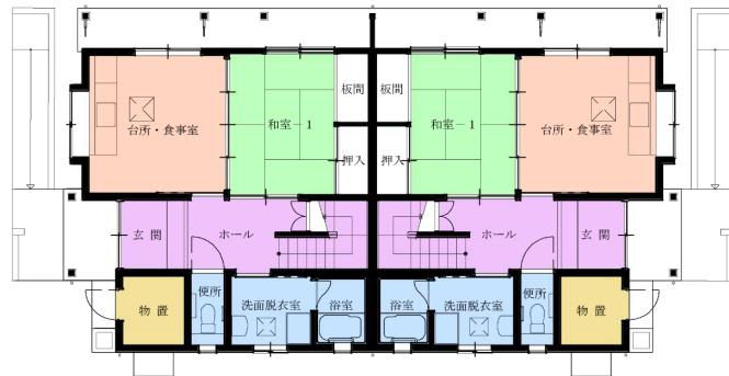
2階建 1階平面図
