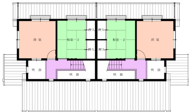
2階建 2階平面図
